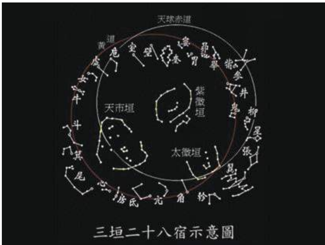
天星三垣廿八宿示意圖
